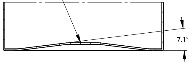
A-A (1 : 7)
